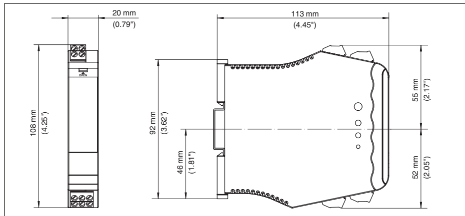
Fig. 2: Dimensões VEGATRENN 152
