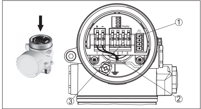
Res. 16: Elektronik bölgesi - İki hücreli gövde
