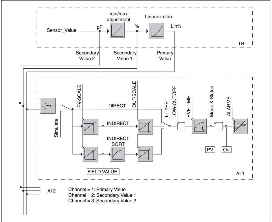
Res. 29: VEGACAL 69 ölçüm değerli işlem
