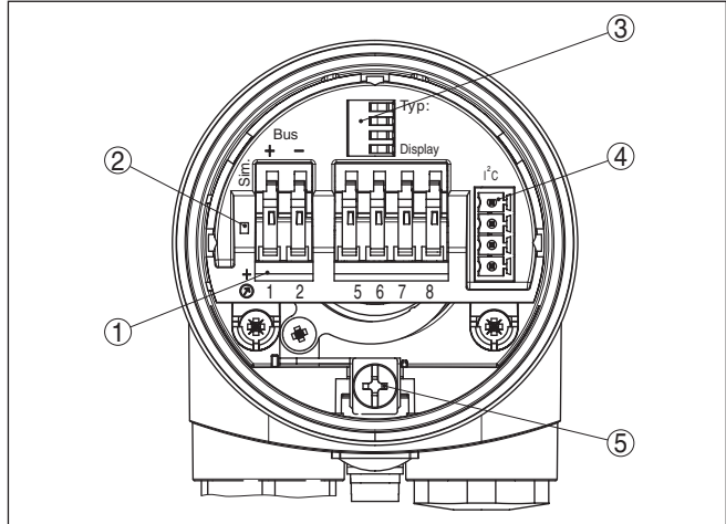
Res. 9: Tek hücreli gövdede elektronik ve bağlantı bölgesi
