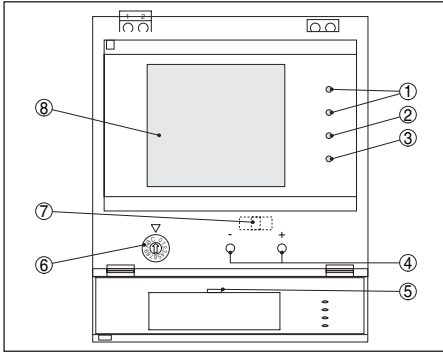
Abb. 25: Éléments de réglage et d'affichage
