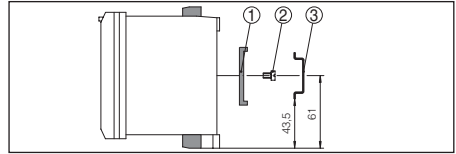
Abb. 4: Tragschienenmontage
