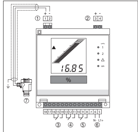
Abb. 33: Esquema de conexión con sensor de dos hilos
