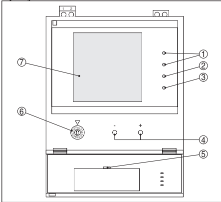
Abb. 19: VEGAMET 381 Ex
