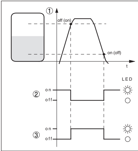
Abb. 26: Modes de fonctionnement des relais
