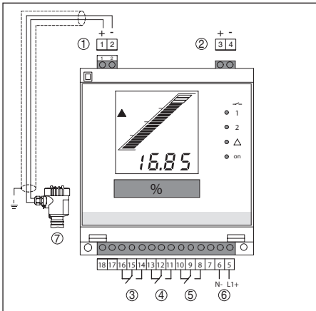
Abb. 6: Anschlussplan mit Zweileitersensor
