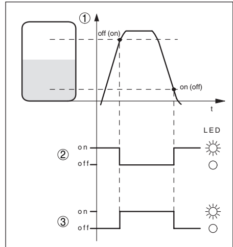
Abb. 8: Relaisbetriebsarten
