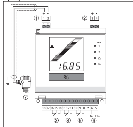
Abb. 24: Schéma de raccordement avec capteur bifilaire
