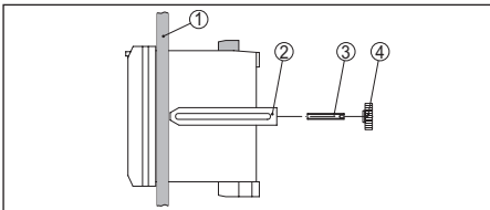
Abb. 2: Schalttafeleinbau
