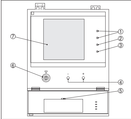
Abb. 1: VEGAMET 381 Ex
