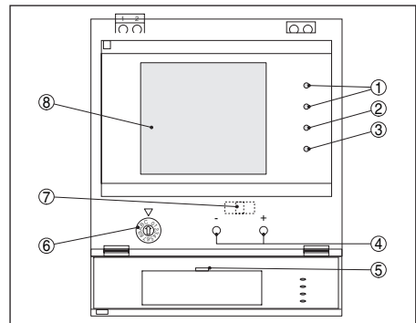
Abb. 7: Anzeige- und Bedienelemente
