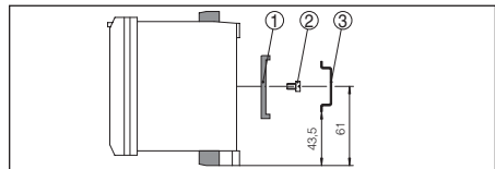
Abb. 22: Montage sur rail
