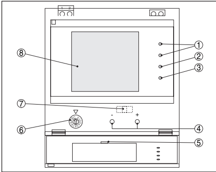
Abb. 34: Elementos de indicación y ajuste
