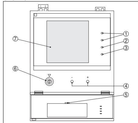
Abb. 10: VEGAMET 381 Ex
