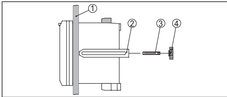
Abb. 29: Montaje en panel de control
