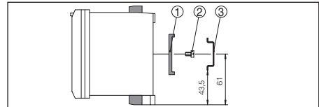
Abb. 31: Montaje en regleta
