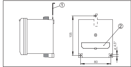
Abb. 30: Montaje con tornillo
