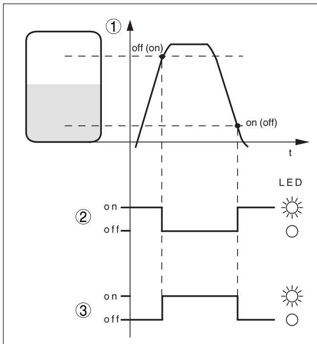
Figura 8: Funzioni a relé
