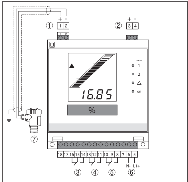
Figura 6: Schema elettrico con sensore bifilare
