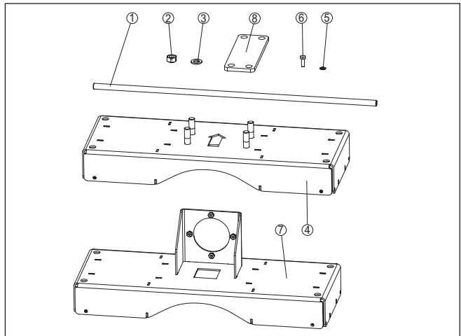
Figura 2: Dispositivo di montaggio KV 31 per tubi a irraggiamento perpendicolare - montaggio verticale del sensore
