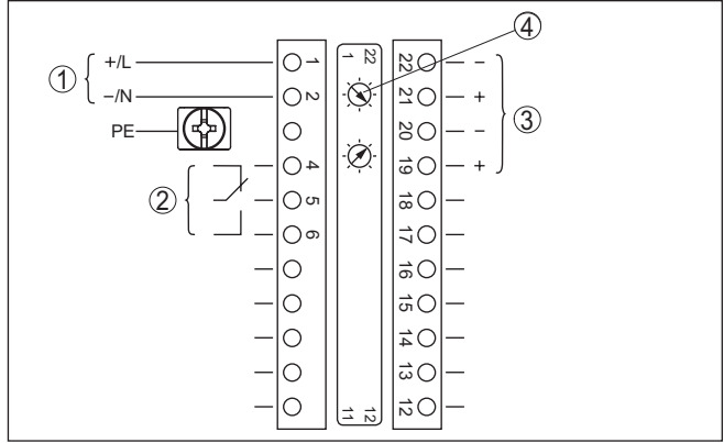
Res. 13: Bünyesinde güvenliği olan akım çıkışlı cihazlarda elektronik bölme ve bağlantı bölümü (Ex d)
